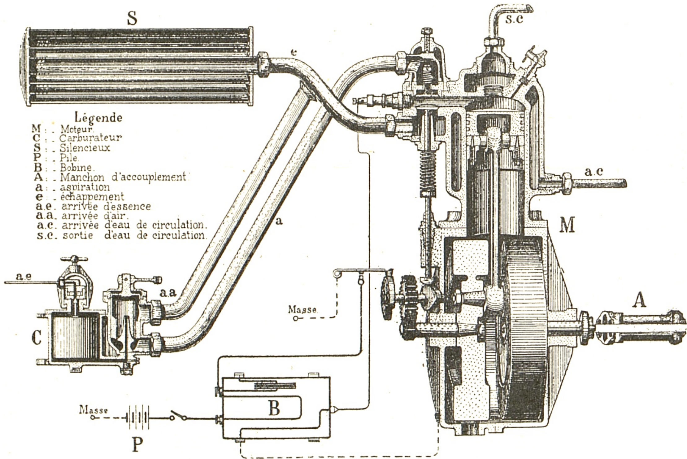
Schéma du système moteur de la petite Voiture
