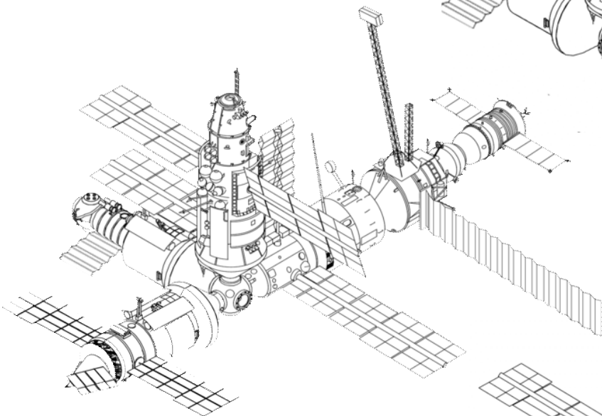
Spektr docks Jun. 1, 95
