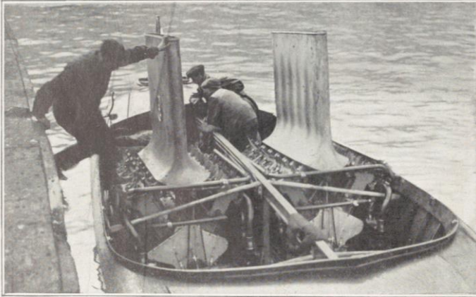
LES MOTEURS DU " PANHARD-TELLIER II " Le " Panhard-Tellier II " est actionné par un moteur 24 cylindres de 1.400 chevaux. L'échappement se fait par deux cheminées latérales. C'est l'excellent sportsman Emile Dubonnet, qui conduit ce splendide canot.
